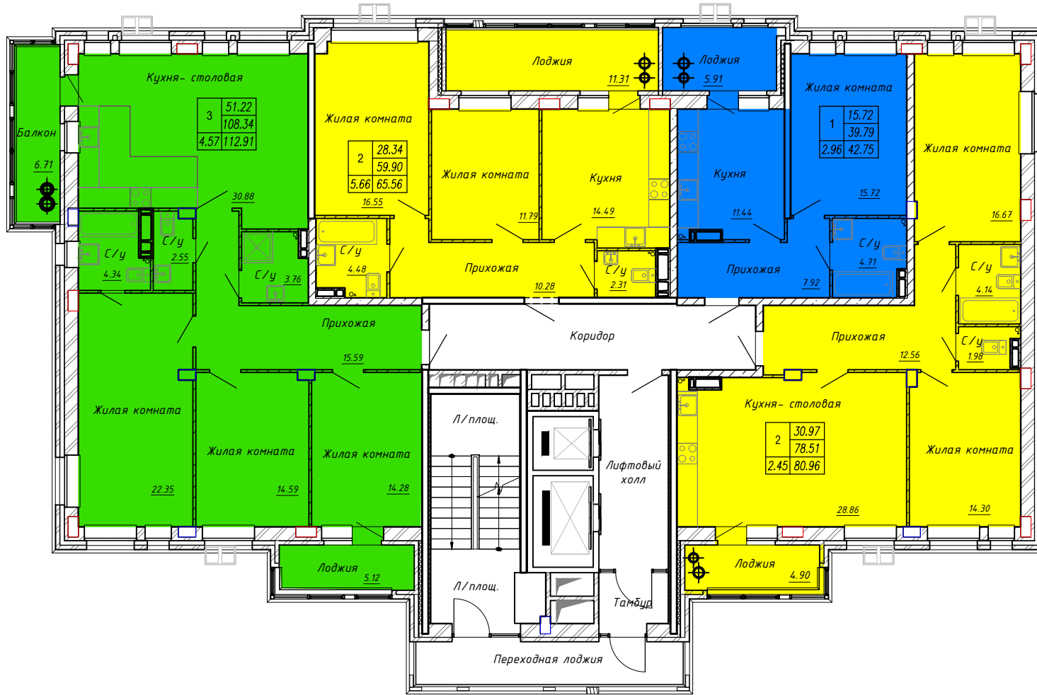
План 9, 10 этажа
