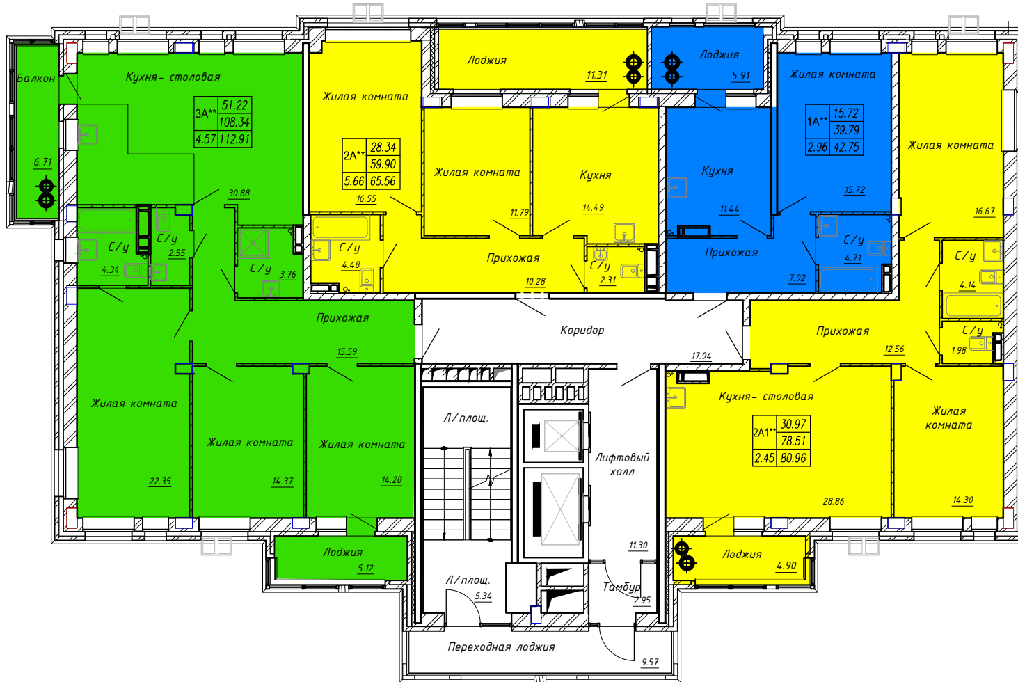
План 13, 14 этажа
